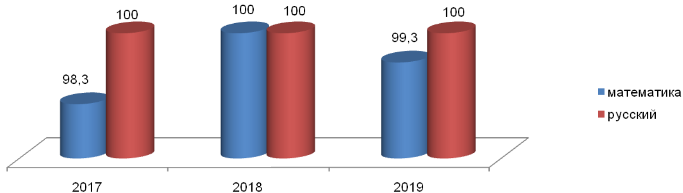
Успешность (%)
